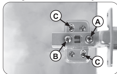
Fig. 2-2 Adjust door
