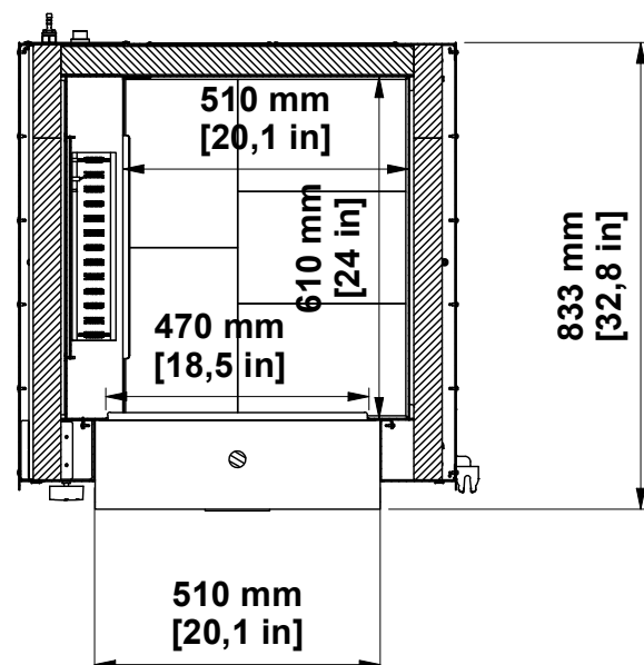
A-A (1 : 15)
